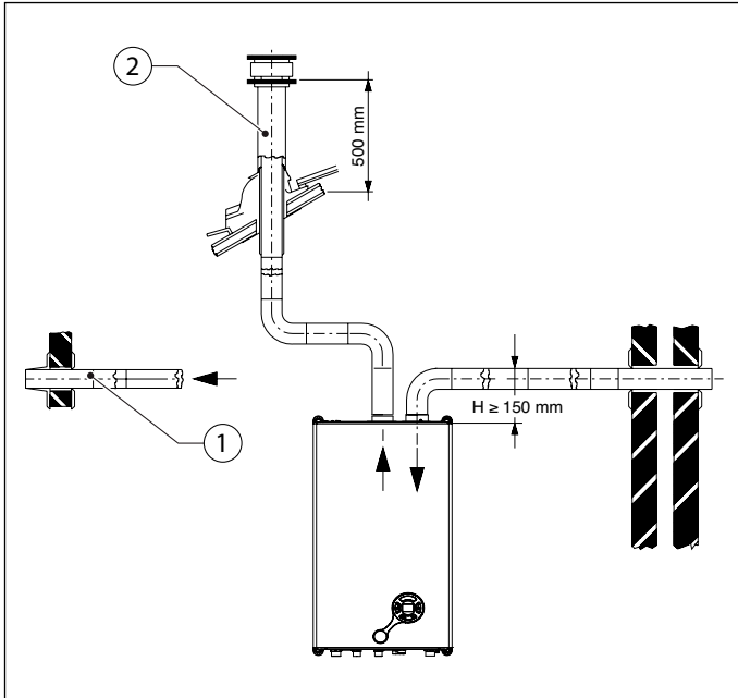
Рис. 14 Приклади системи забору повітря/викиду продуктів згоряння
