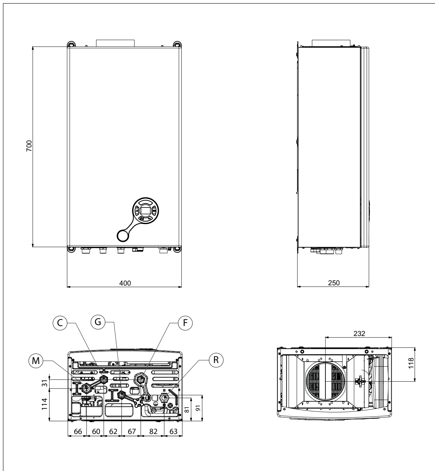
Рис. 4 Габарити CTN
